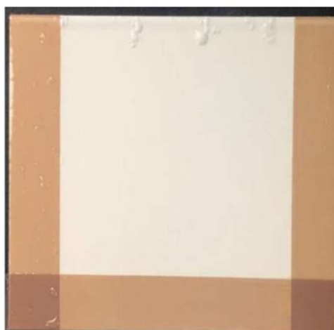
氟碳板表面出现起泡现象 涂层有脱落风险
