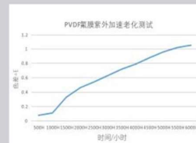
测试依据紫外老化 (GB/T16422.3-2014)
